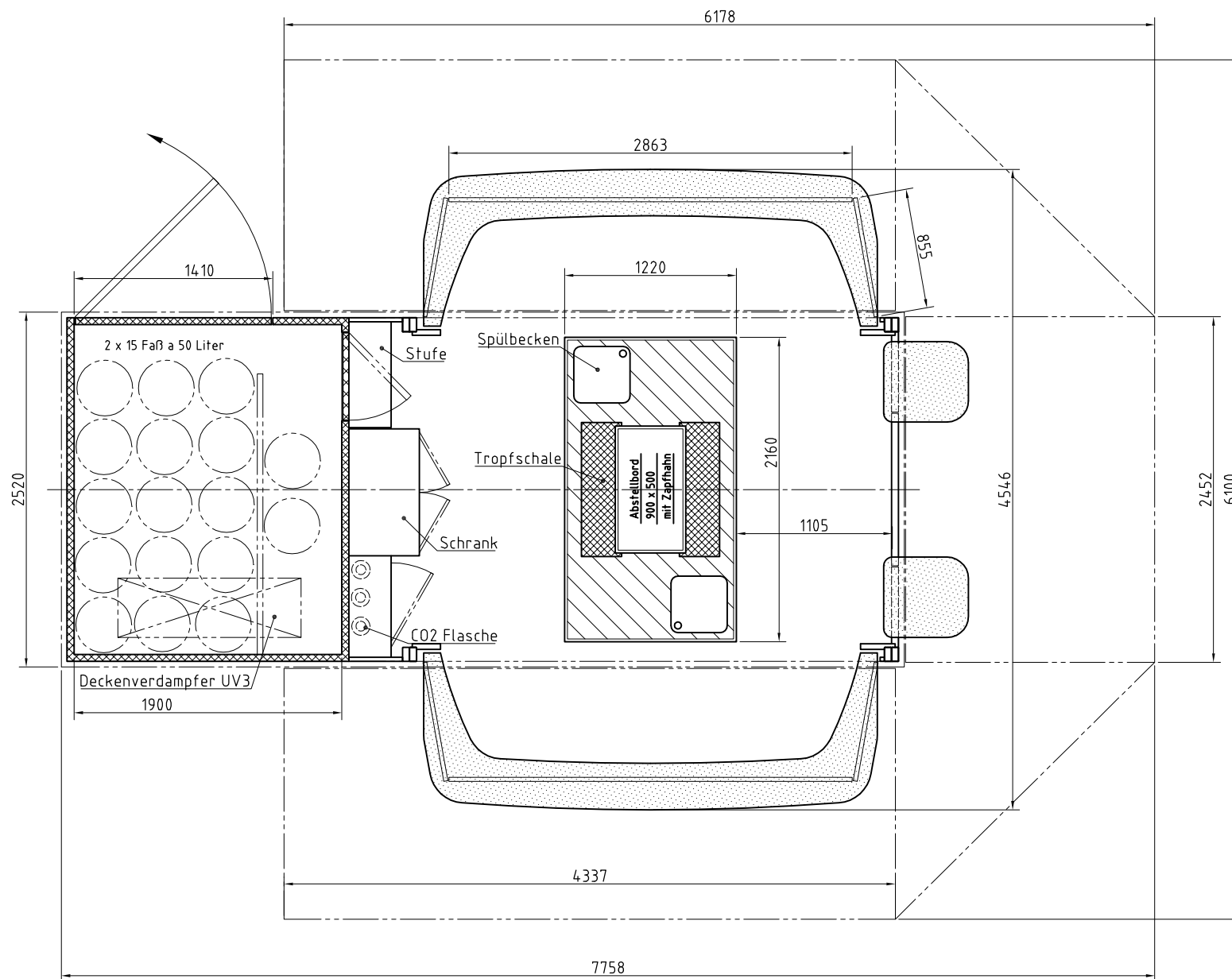
Grundrisszeichnung APK-2
